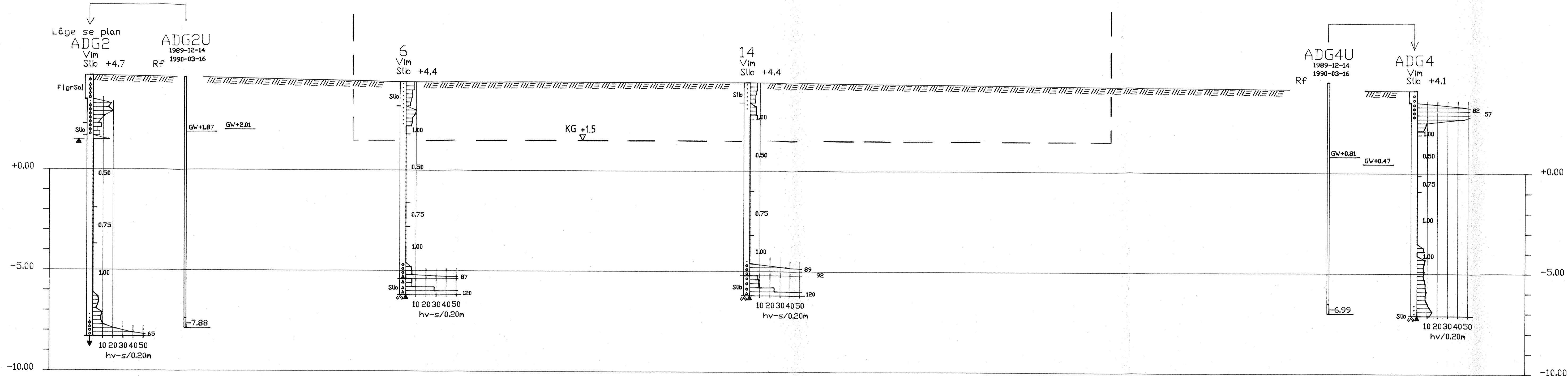
SEKTION F-F 1: 100
