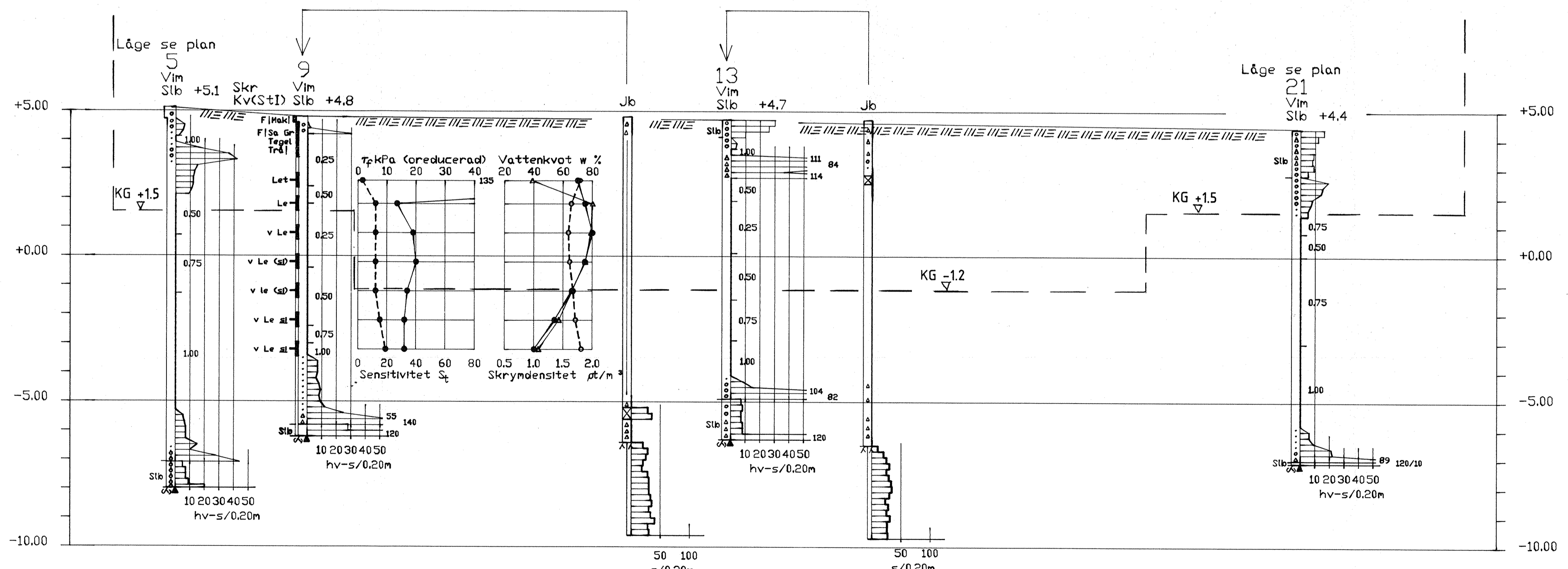
SEKTION G-G 1: 100
